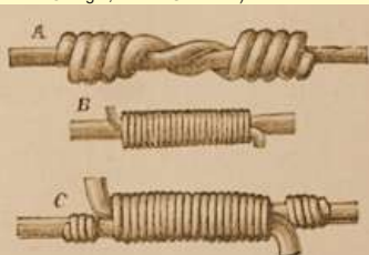
Empalme de cables eléctricos en 1892 (Manuel pratique de l'installation de la lumière électrique. Installations privées, de J.-P. Anney)
